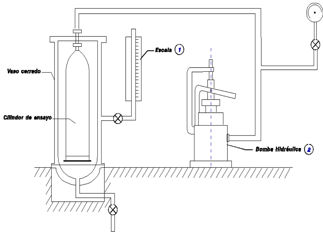
PRUEBA DE HERMETICIDAD FIG. 4
