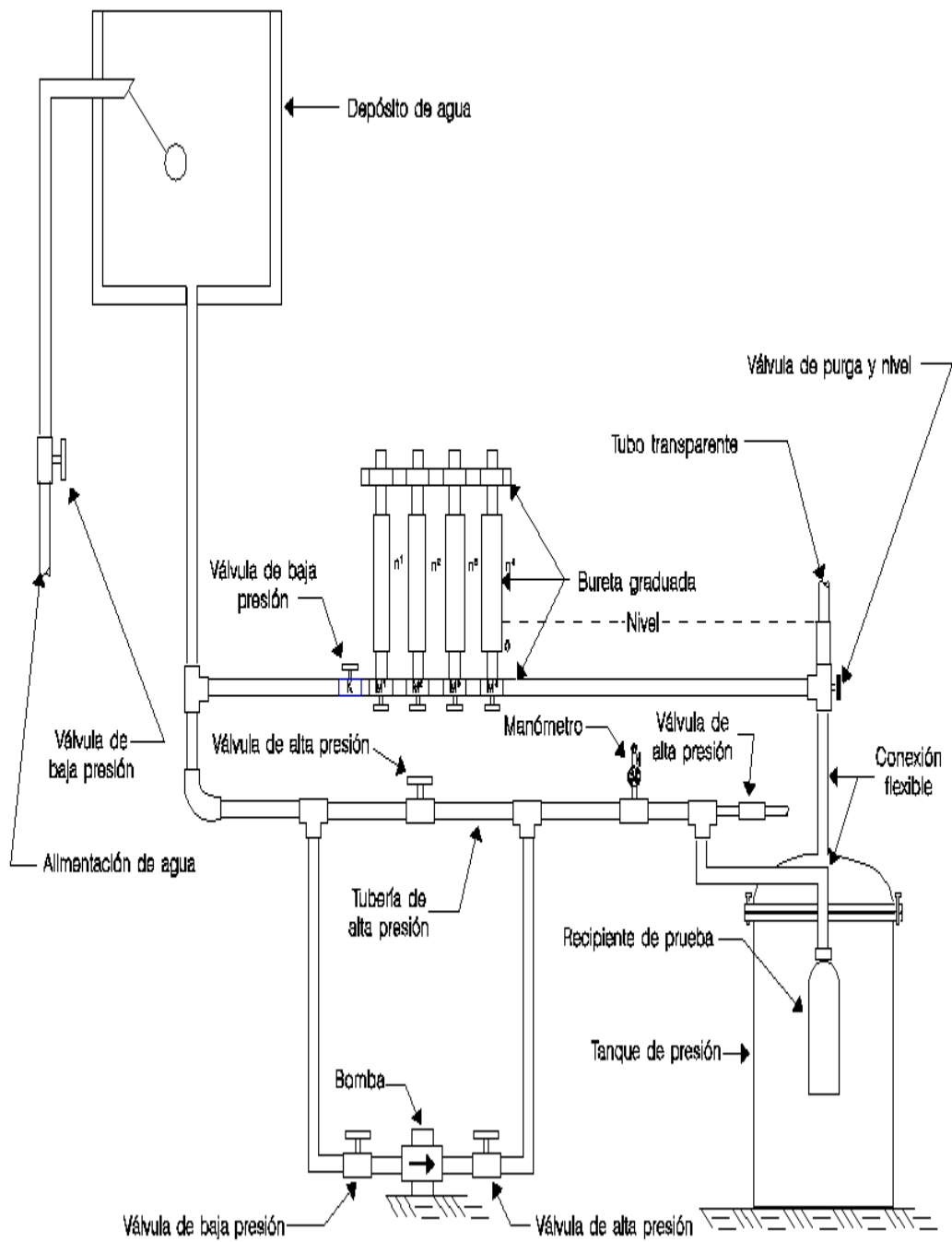
PRUEBA DE RUPTURA FIG. 3
