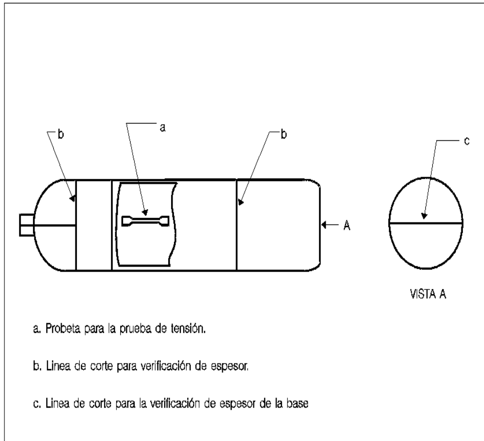
PRUEBA DE DEFORMACION PERMANENTE FIG. 2
